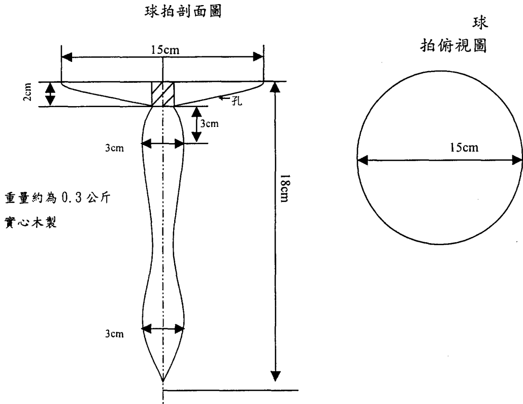
圖三 Turul 運動球拍的規格圖
