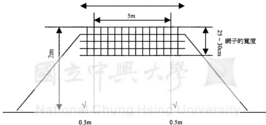
圖二 Turul 運動球網的規格圖
