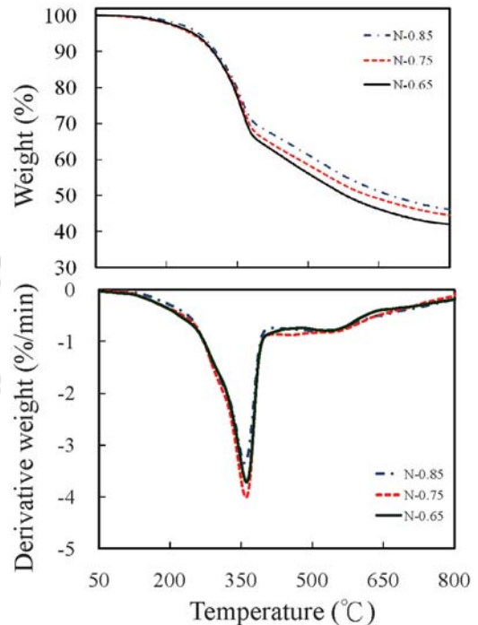
圖5. PF樹脂成型板之TG及DTG曲線圖
